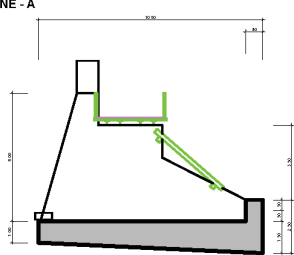
SEZIONE - A
