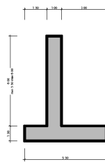
SEZIONE - D
