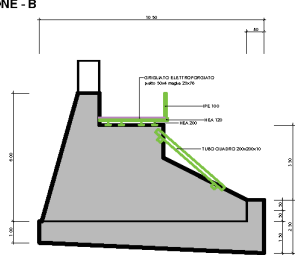
SEZIONE - B
